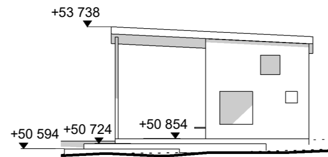
RAK2 Julkisivu lounaaseen 1:100
