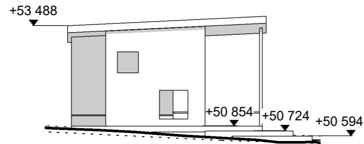
RAK2 Julkisivu luoteeseen 1:100
