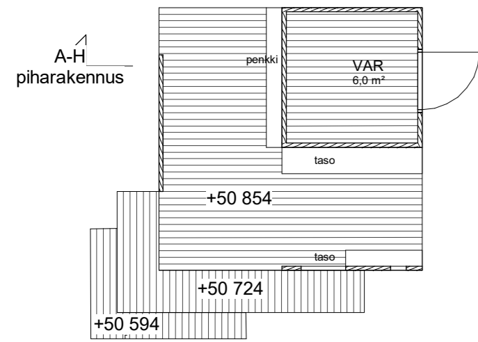
RAK2 Pohjapiirros 1:100
