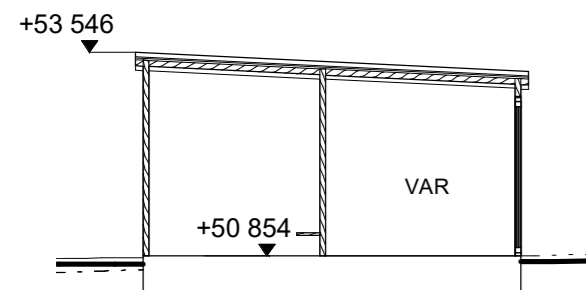
RAK2 Leikkaus A-H 1:100
