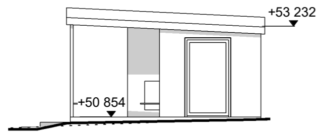
RAK2 Julkisivu kaakkoon 1:100
